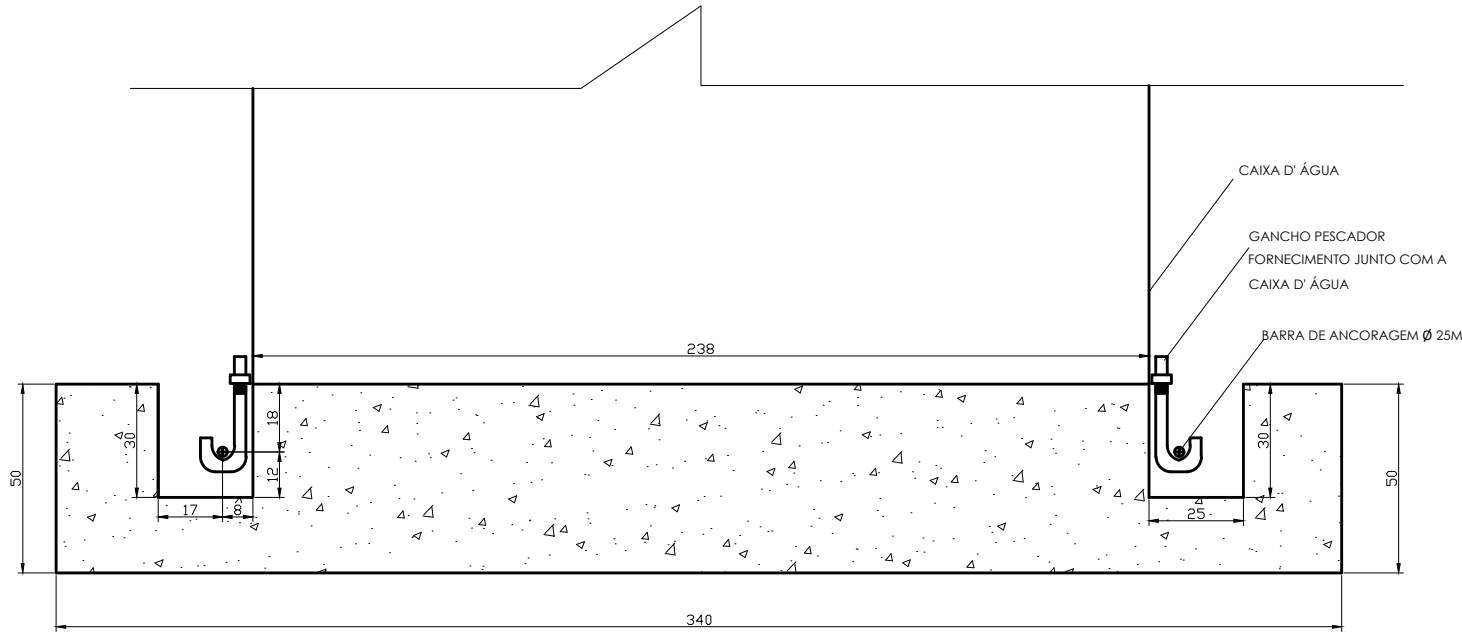
DETALHE DA FIXAÇÃO DA CAIXA D' ÁGUA ESCALA:1:20
