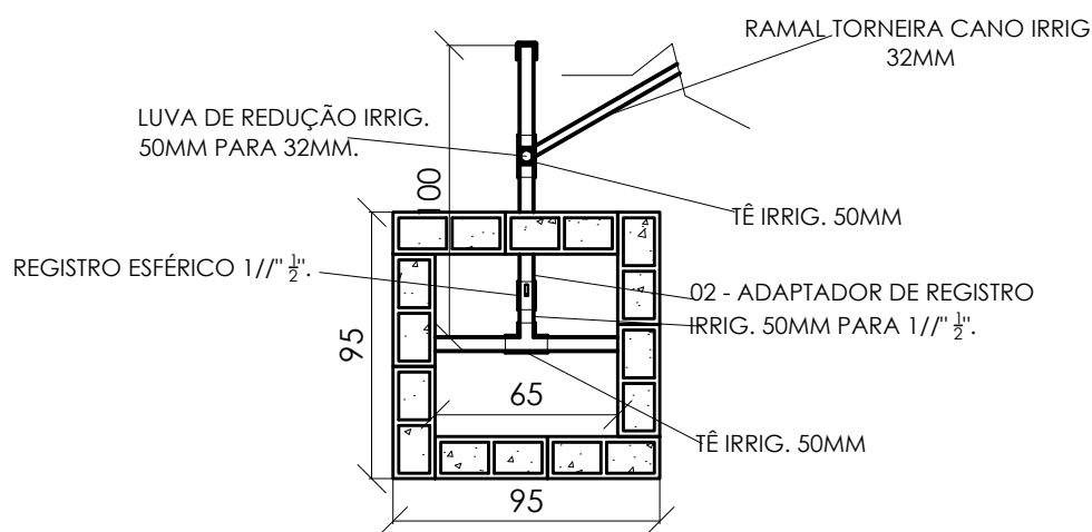
DETALHE CAIXAS DE PASSAGENS ESCALA:1:30
