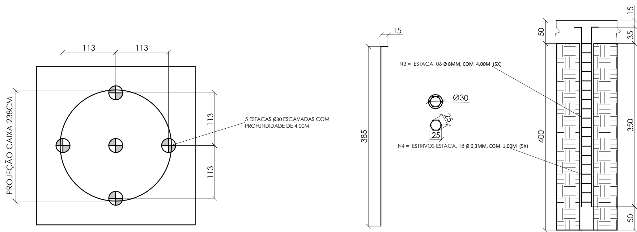
DETALHE DA FIXAÇÃO DA CAIXA D' ÁGUA ESCALA:1:20
